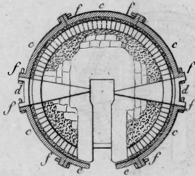
Coupe horizontale à la hauteur de C D.
