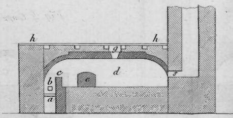
Fig. 2. Coupe suivant A B.
