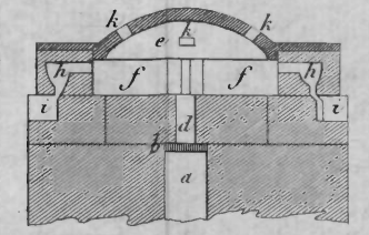
Fig. 7. Coupe suivant G H.
