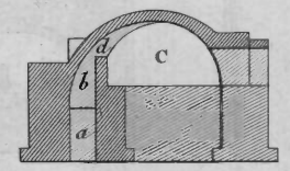
Fig. 4. Coupe suivant C D.
