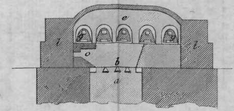
Fig. 6. Coupe suivant E F.
