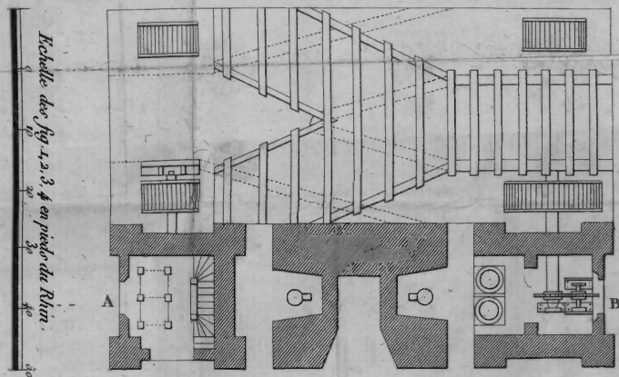
Fig. 1. Plan de l'Usine de Malapane.
