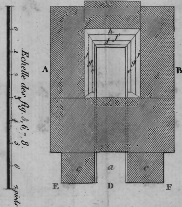
Fig. 5. Plan de l'ouvrage.
