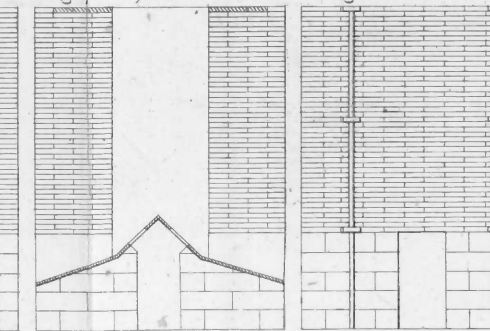
Fig. 6. Coupe transversale.
