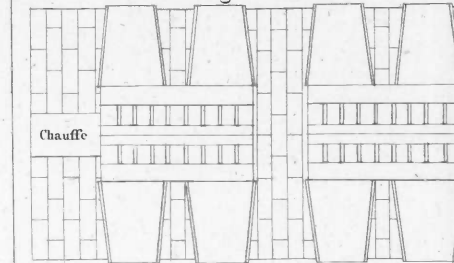
Fig. 4. Coupe transversale.
