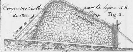
Moule de carbonisation à bois couché
