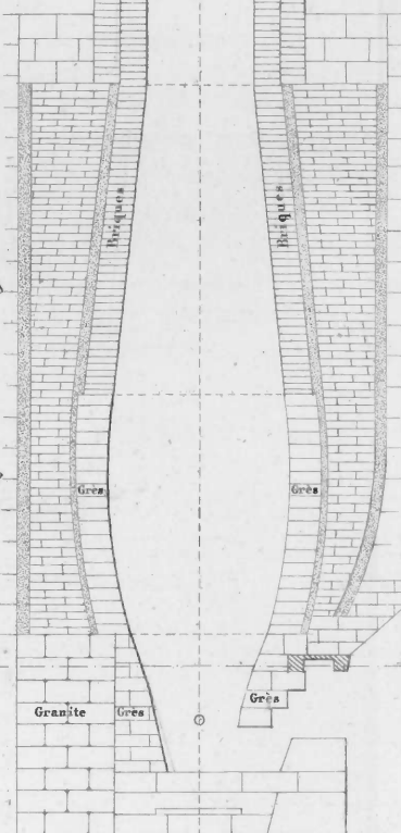
Fig. 14. Coupe horizontale par la ligne AB de la Fig. 15
