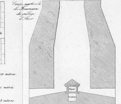
Fig. 7. Coupe verticale.
