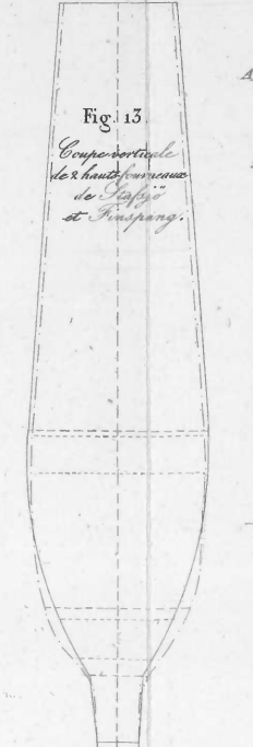
Fig. 13. Coupe verticale de 2 haut-fourneaux de Stajfjé et Finspang
