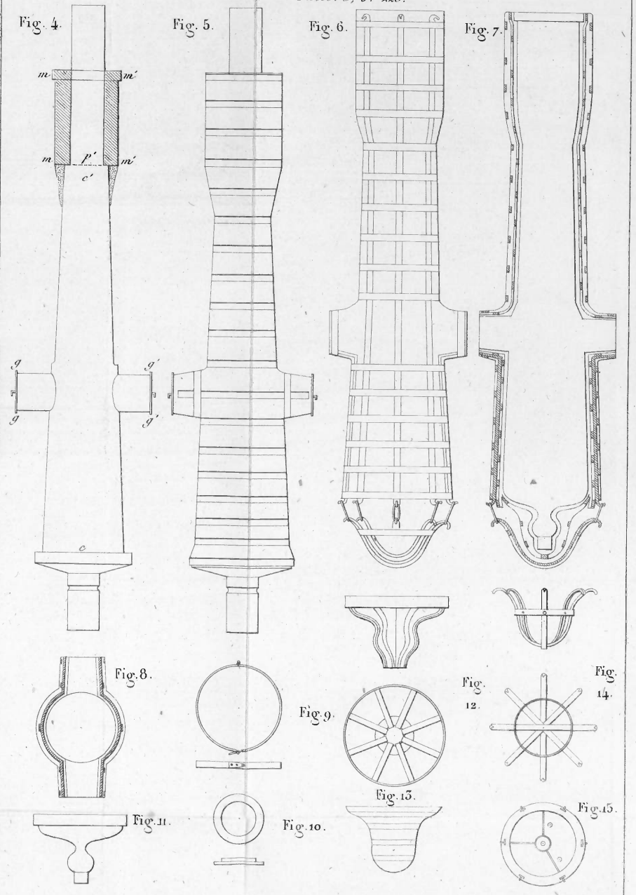
Détails du Moulage d'un Obusier danois de 84 — Calibre, 0 m 228.
