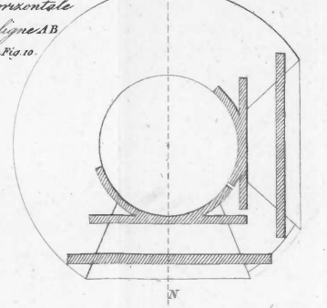
Fig. 10. Coupe verticale par la ligne MN de la Fig. 9
