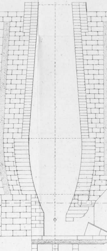
Fig. 9. Coupe horizontale par la ligne AB de la Fig. 10
