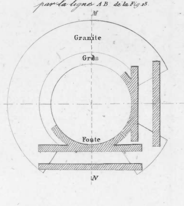
Fig. 14. Coupe horizontale par la ligne AB de la Fig. 15
