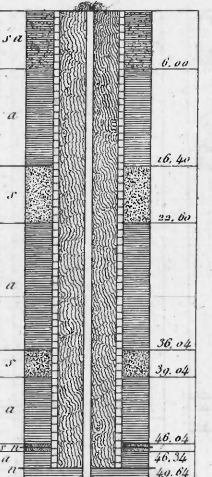
Sondage de Kébour oued rior. Fig. 5.
