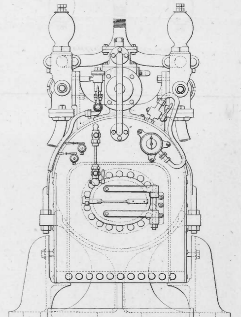
Fig. 7. Coupe C.D.
