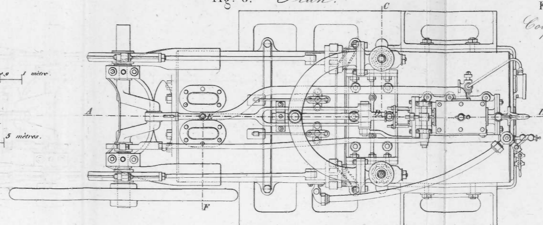
Fig. 6. Plan.
