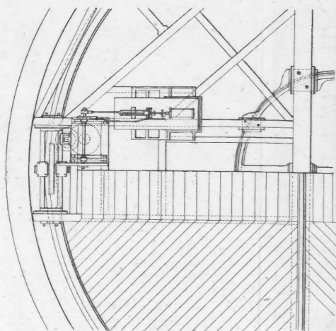
Fig. 2. Plan.
