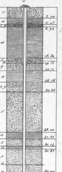
Sondage de Camerna. Fig. 8.
