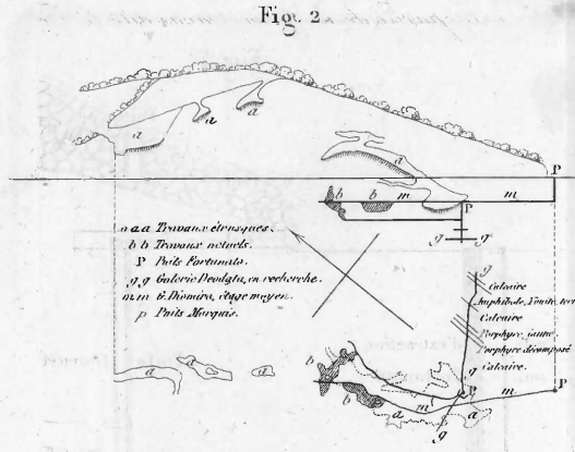
Disposition en Plan des anciens travaux (Mine de Campiglia)
