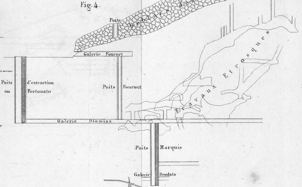
Plan et Coupe de la partie des travaux anciens encore accessibles aux mines des Rocchette près la Viciolletta.
