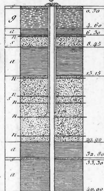
Sondage de Chegga. Fig. 7.
