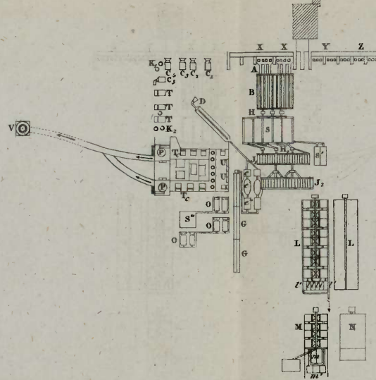
Fig. 3. Partie de l'Atelier de S. Day Unital. 1857.
