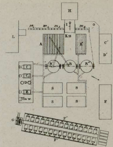
Fig. 2. Partie de l'Atelier de Timorft. 1857.
