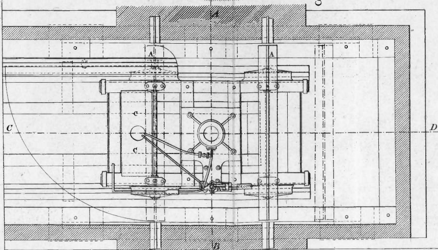
Fig. 8. Plan.
