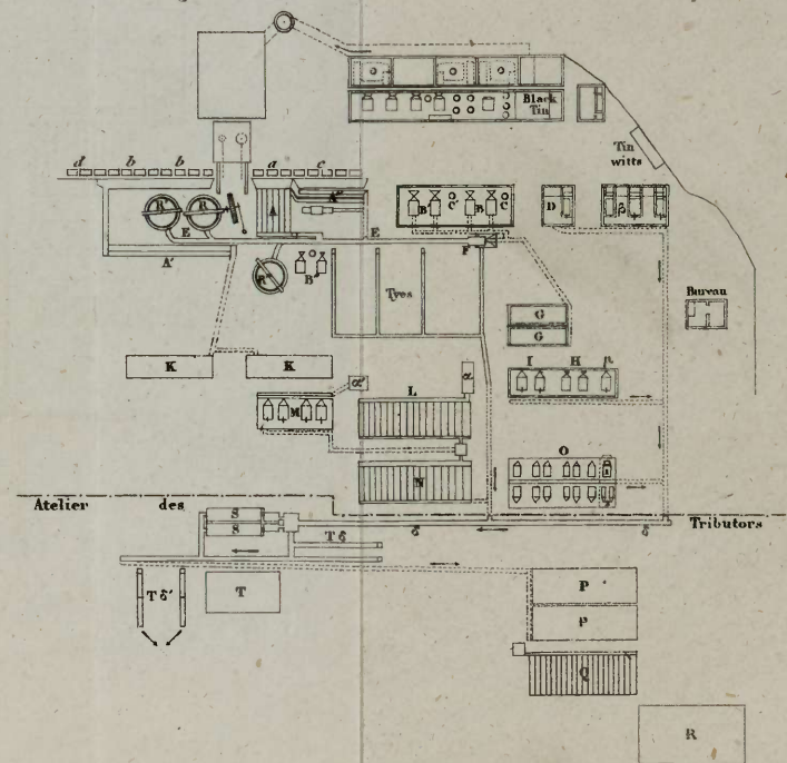
Fig. 4. Atelier de Par Consols. 1857.
