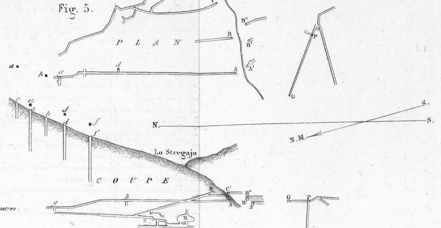
Plan et Coupe de la partie des travaux anciens encore accessibles aux mines des Rocchette près la Viciolletta.
