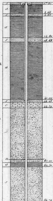
Sondage de Chegga. Fig. 7.
