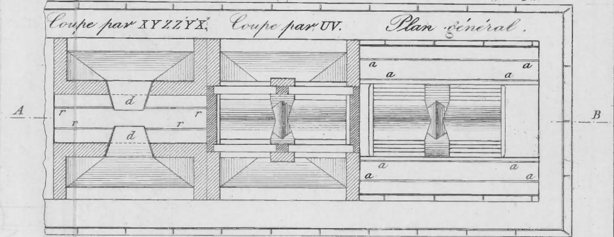
Coupe transversale d'une double rangée de fours.
